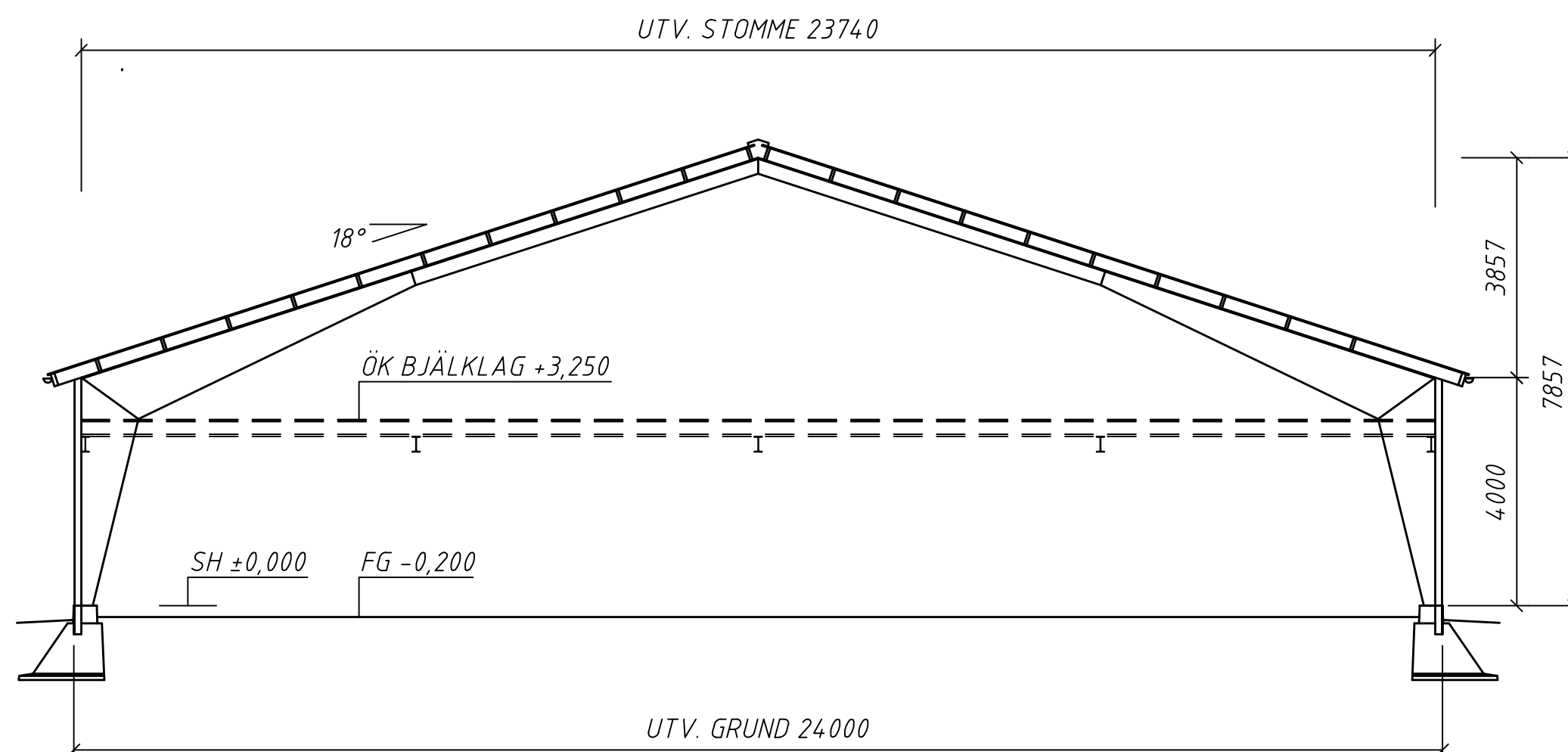
SEKTION -1:100-
